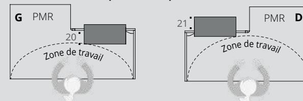
Parement sans entretoise Vue de dessus
