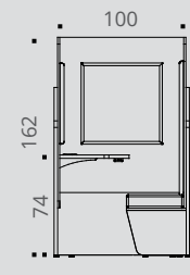
Cabine assise avec banc tablette à gauche vue de face
