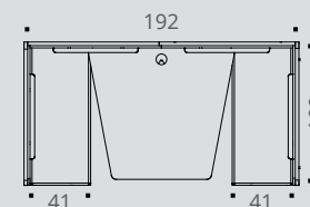
Cabine assise Duo avec bancs vue de dessus
