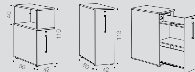
Caisson Tower avec Top box H 110 cm
