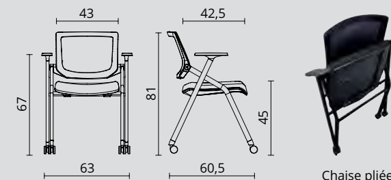
Chaise pliée
