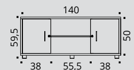
Console B-box 2 portes coulissantes H 59,5 cm
